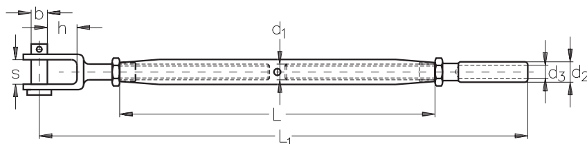
ASS Super-Mini-Ridoir à chape filetée à gauche et terminaison, cage longue
