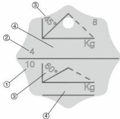
Marquage pour élingue chaîne multibrins
