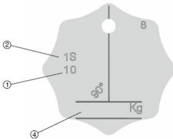
Marquage pour élingue chaîne 1 brin
